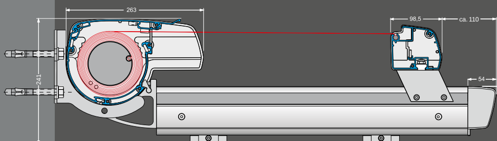
Capri type Dakmontage
