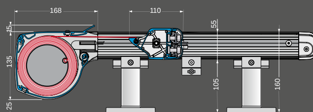
Ancona type Bovendak
