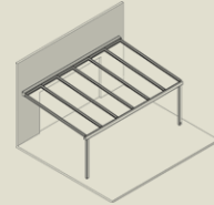
B1 bündig, Pfosten außen B1s wie B1, mit Stahlverstärkung
